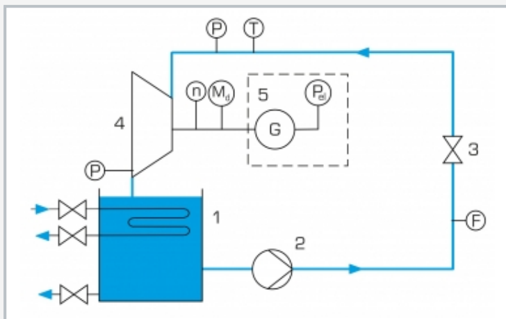
1 depósito con refrigeración opcional, 2 bomba centrífuga, 3 válvula de estrangulación, 4 turbina Francis, 5 generador; P presión, T temperatura, F caudal, n número de revoluciones, M_d par, P_e potencia eléctrica
