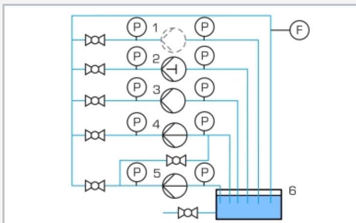
Esquema del proceso 1 puesto libre para bomba adicional (disposición del usuario), 2 bomba de émbolo, 3 bomba de canal lateral, 4+5 bombas centrífugas, 6 depósito; F caudal, P presión
