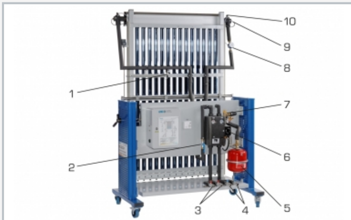
1 Druckaufnehmer, 2 Absperrventil, 3 Anschlüsse für Warmwasser, 4 Anschlüsse für Kaltwasser, 5 Membranausdehnungsgefäß, 6 Pumpe, 7 Überdruckventil, 8 Durchflusssaufnehmer, 9 Temperatureaufnehmer, 10 Entlüftungsventil
