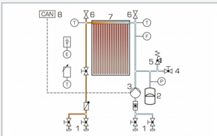
1 Anschlüsse für Wärmeträgerleitungen mit Absperrventilen und Schnellkupplung, 2 Membranausdehnungsgefäß, 3 Pumpe, 4 Befüllventil, 5 Überdruckventil, 6 Entlüftungsventile, 7 Vakuümrohrenkollektor, 8 CAN-Bus; E Beleuchtungsstärke, F Durchfluss, T Temperatur, P Druck
