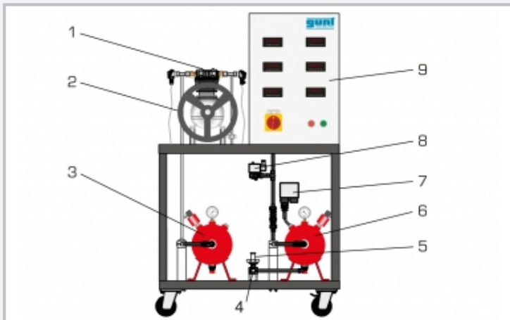
1 compresseur, 2 poulie de courroie, 3 réservoir d'aspiration, 4 soupape de purge avec silencieux, 5 soupape de sécurité, 6 réservoir sous pression, 7 pressostat, 8 électrovanne, 9 armoire de commande avec affichages numériques
