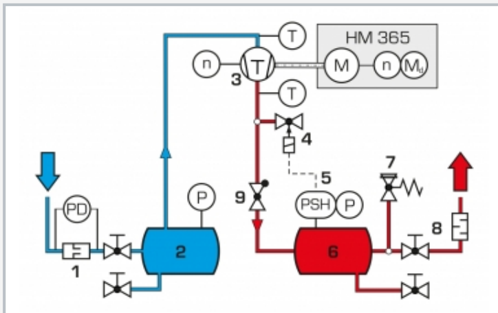
1 tuyère de mesure, 2 réservoir d'aspiration, 3 compresseur à piston, 4 électrovanne, 5 pressostat, 6 réservoir sous pression, 7 soupape de sécurité, 8 soupape de purge avec silencieux, 9 soupape de retenue; P pression, PD pression différentielle, T température, n vitesse de rotation, M_1 couple
