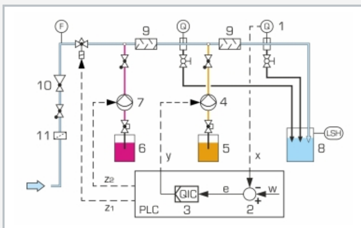
1 élément de mesure: capteur de pH intelligent, 2 comparateur: composant de l'API, 3 régulateur numérique intégré à l'API, 4 actionneur: pompe de dosage de l'acide, 5 réservoir de produits chimiques pour l'acide, 6 réservoir de produits chimiques pour la base, 7 pompe de dosage de la base, 8 réservoir de produit, 9 mélangeur statique, 10 soupape de réduction de pression, 11 collecteur d'impuretés
