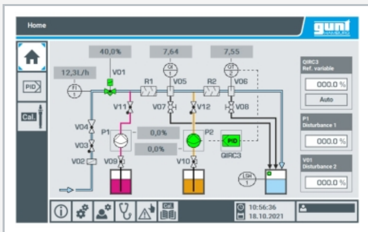
Capture d'écran de l'API: page de démarrage avec schéma de processus et toutes les valeurs mesurées actuelles
