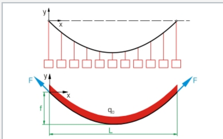
Modelo de un puente colgante: "cable colgante con carga de línea" con diagrama de sólido libre (abajo); F esfuerzo en el cable, q_0 carga de línea; f flecha máxima, L luz
