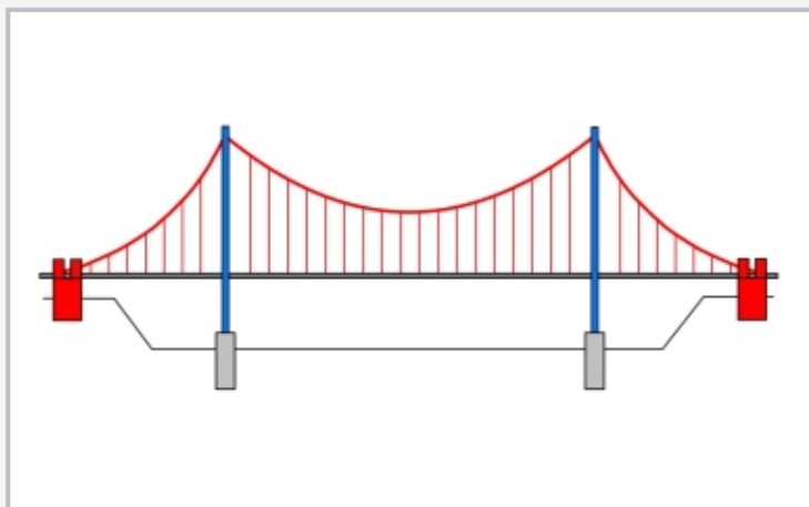
Esfuerzos en un puente colgante: rojo: esfuerzos de tracción (actúan en los cables de sustentación, los ganchos y los anclajes de los cables de sustentación), azul: esfuerzos de compresión (actúan en los pilones)
