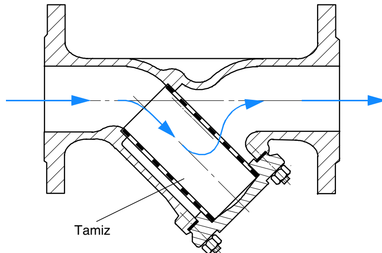
Fig. 4.15 Colector de fango
